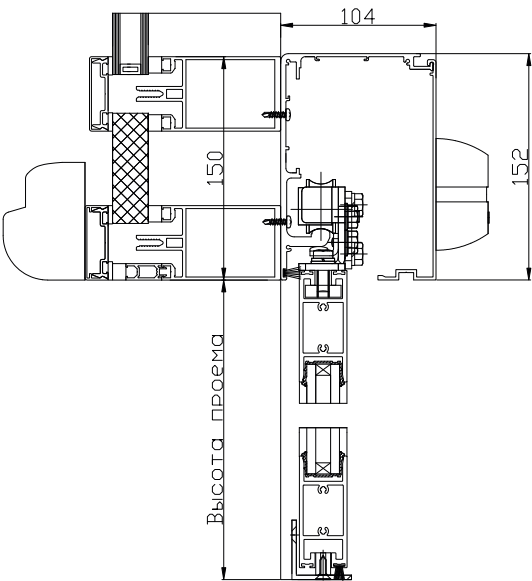
Разрез двери с профилем «ЭНТЕК»
