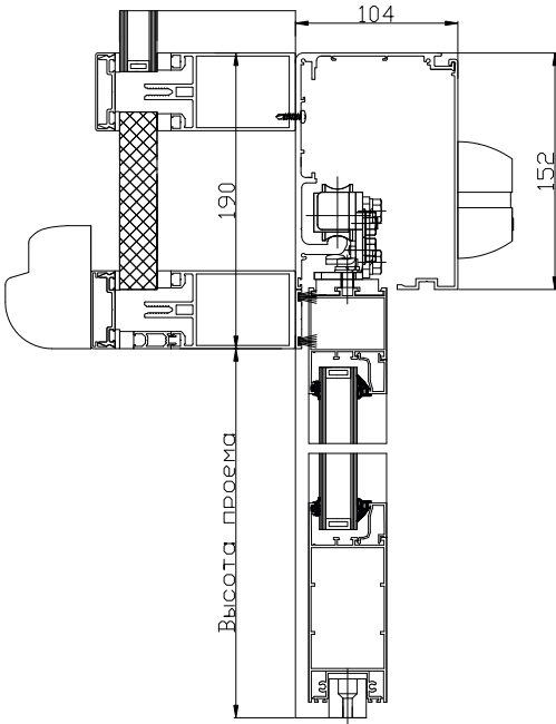
Разрез двери с профилем «РЕАЛИТ»
